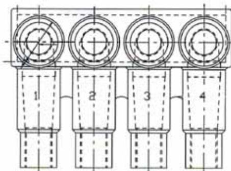
Tipo ISB185-L distância entre saídas = 38 mm
