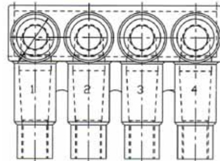
Tipo ISB240-S distância entre saídas = 35 mm
