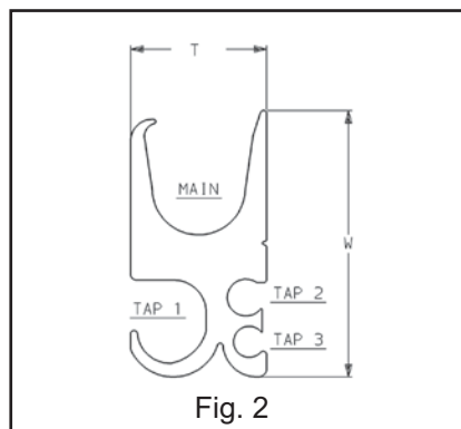
TAP: DERIVAÇÃO - MAIN: PRINCIPAL
