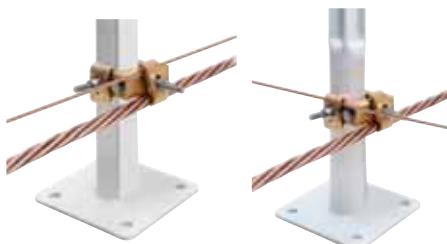
CONFIGURAÇÃO PARALELA
